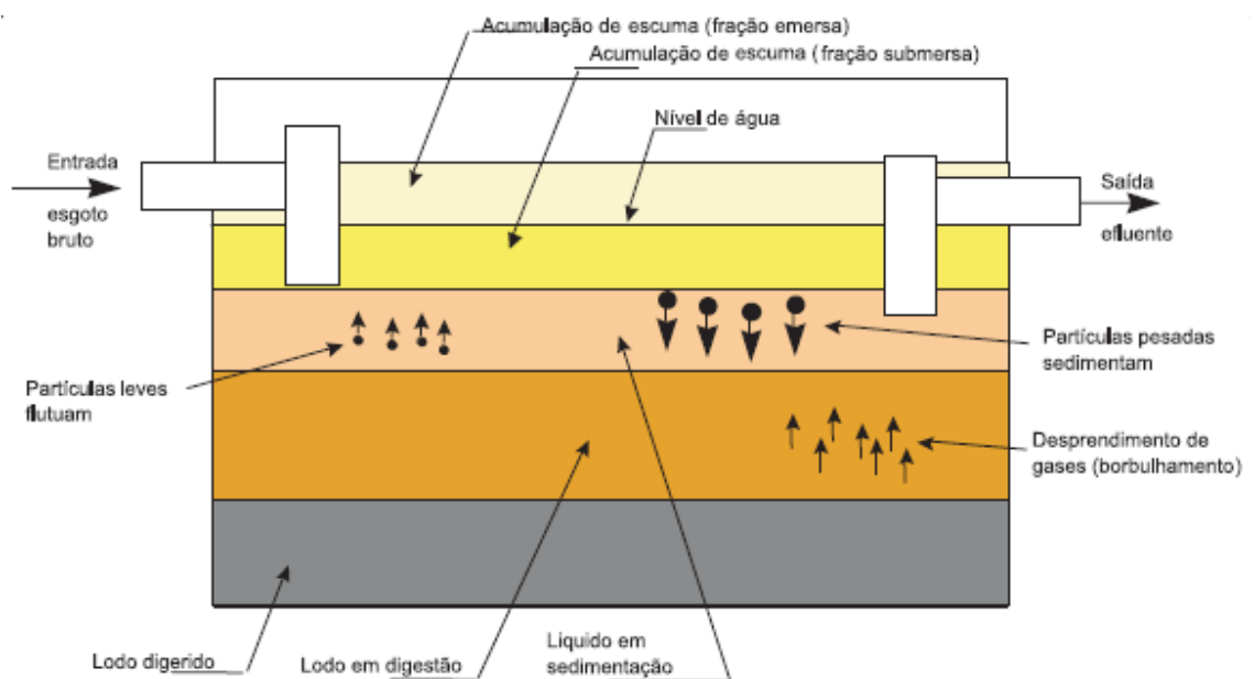
Figura 3– Funcionamento geral de um tanque séptico
