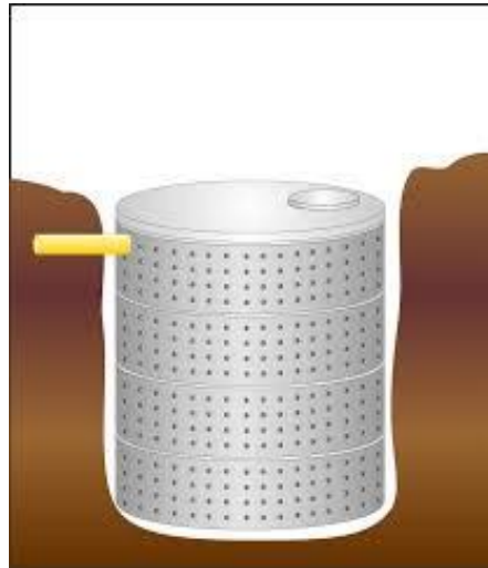
Figura 8 – Tanque de infiltração do esgoto doméstico tratado.
