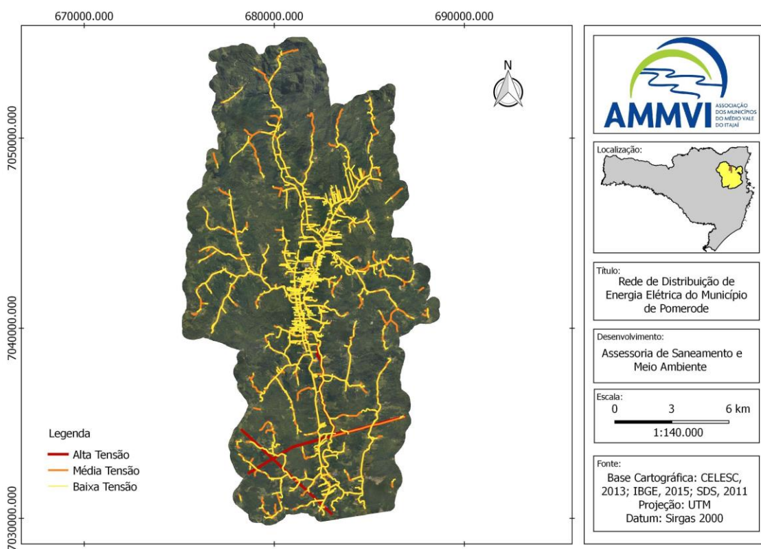
Figura 48 - Rede de Distribuição de Energia Elétrica no Município de Pomerode
