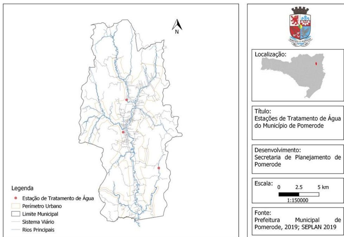
Figura 37 - Estações de Tratamento de Água do Município de Pomerode
