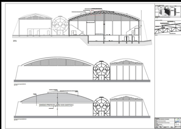
Projeto arquitetônico, prancha 04: corte, elevações e detalhes.
